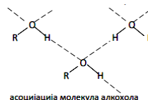
асоцијација молекула алкохола
