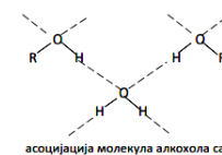
асоцијација молекула алкохола са молекулима воде
