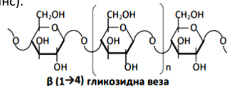
целулоза линеарна структура
