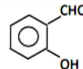
o-хидрокси-бензалдеҳид (салицил-алдеҳид)
