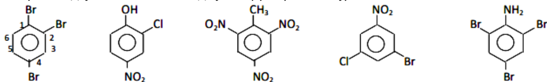
1,2,4-трибром-бензен 2-хлор-4-нитро-фенол 2,4,6-тринитро-толуен 3-бром-5-хлор-нитробензен 2,4,6-трибром-анилин
